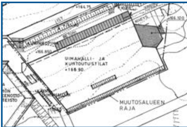
KUVA 71: Uimahallin asemapiirustus vuodelta 1993.
