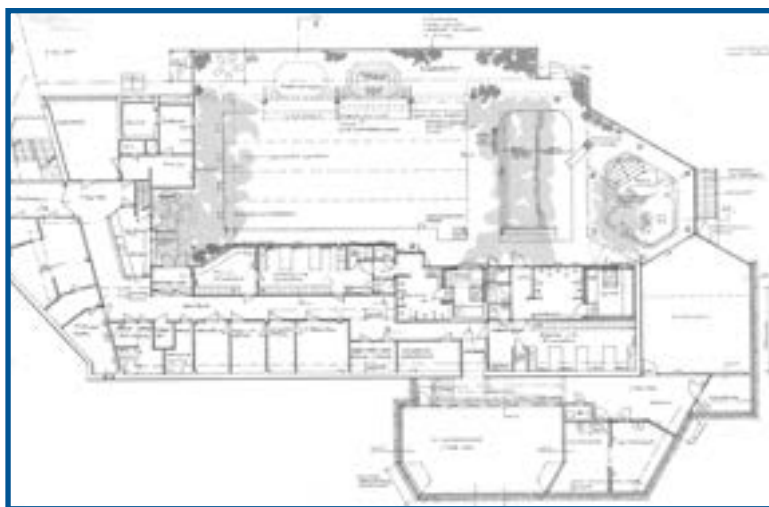
KUVA 68: Uimahallin pohjaluonnos vuodelta 1991.
