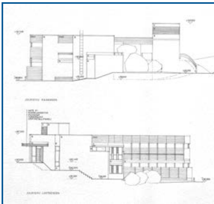
KUVA 59: Arkkitehtitoimiston julkisivupiirustukset vuonna valmistuneesta 1982 lisäsiivestä. Ylempi piirustus kaakosta, alempi luoteesta
