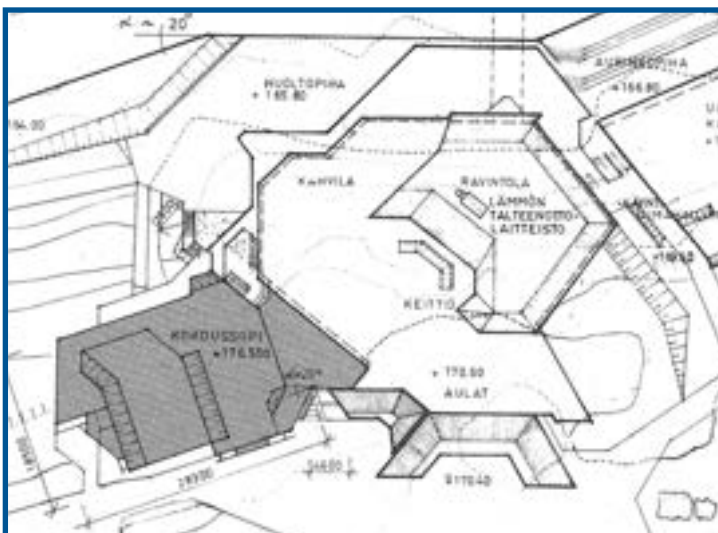
KUVA 77: Kokoussiipilaajennus asemapiirustuksessa.
