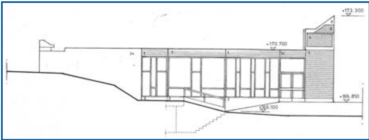
KUVA 70: Uimahallin julkisivupiirustus luoteeseen vuodelta 1993.
