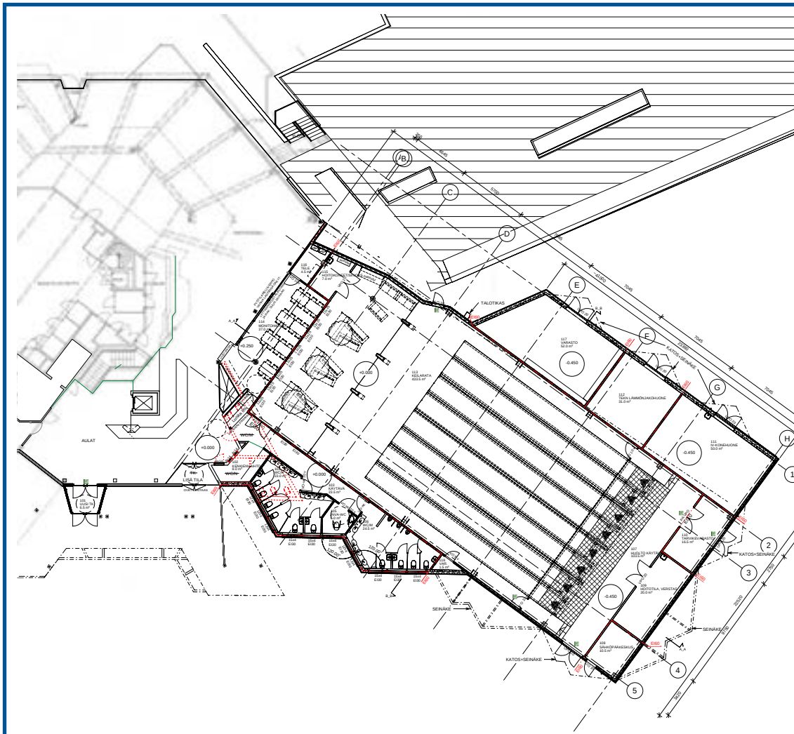
KUVA 83: Motiivi Oy:n pohjapiirustus keilahallista
